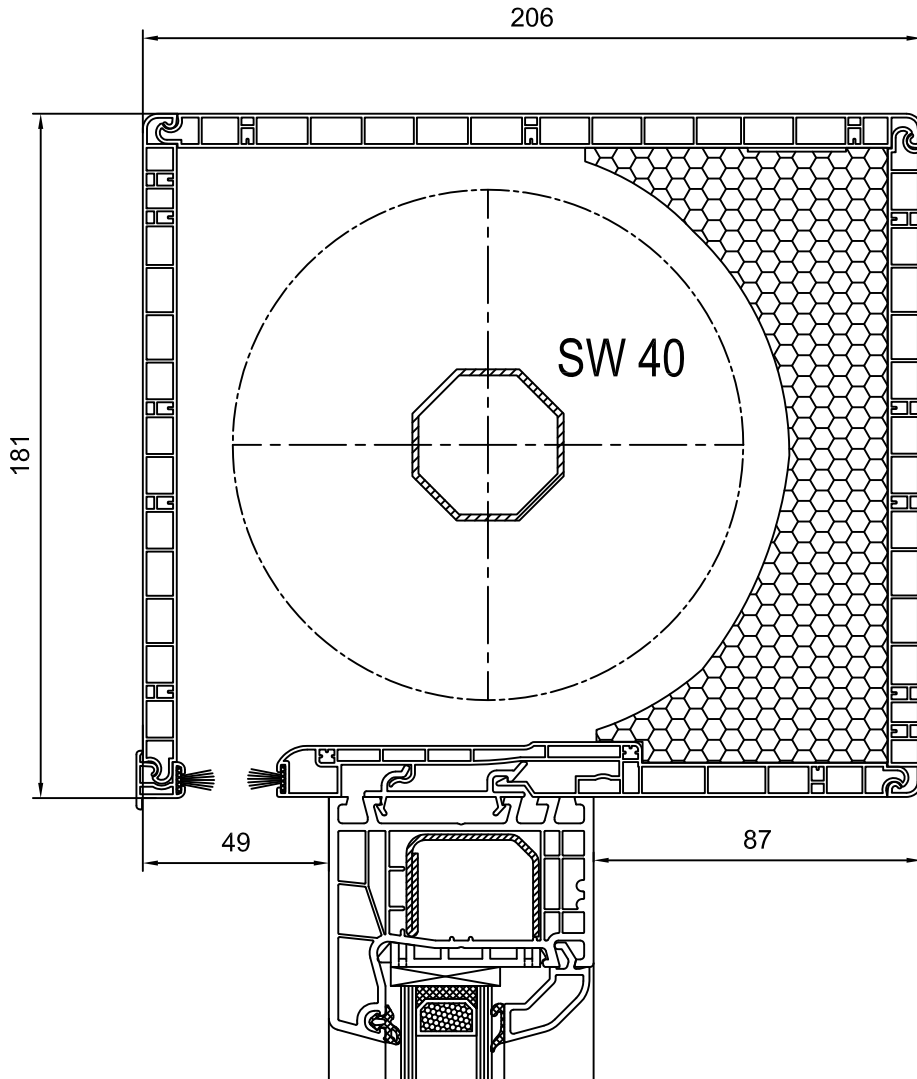
Art.500502 - Rollladenführung (einfach)
