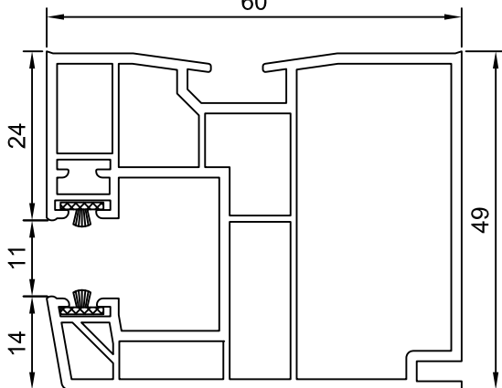
Art.500502 - Rollladenführung (einfach)
