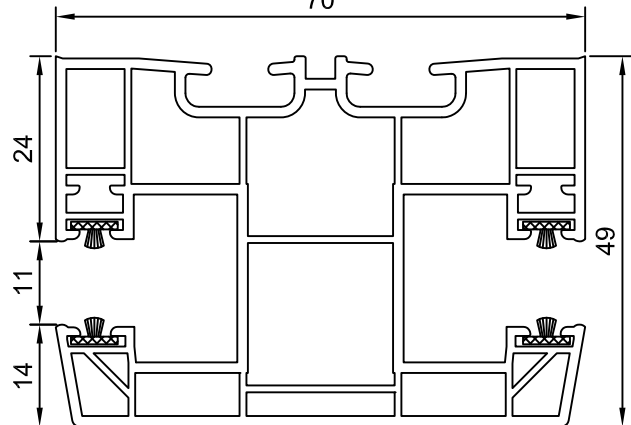
Art.500504 - Rollladenführung (doppelt)
